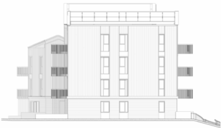
FASADE BYGG A SØR-ØST
